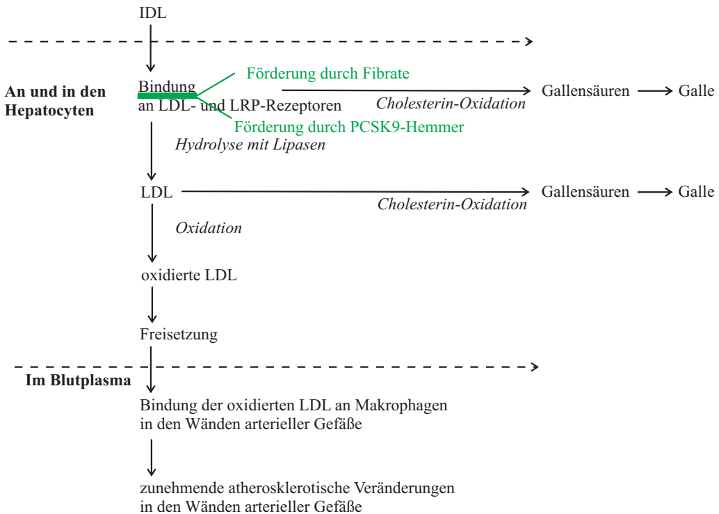
Abb. 32.4: Endstrecke des LDL-Weges.
