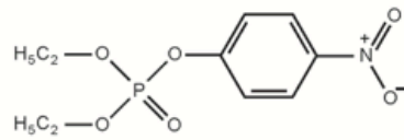
Paraoxon (Pestizid)
