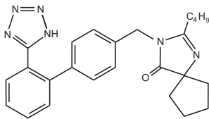
Irbesartan
