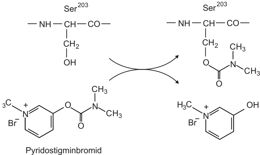
Abb. 63.1. Pyridostigmin reagiert kovalent mit dem Ser203 der Acetylcholinesterase.
