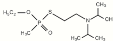
VX (Kampfstoff)
