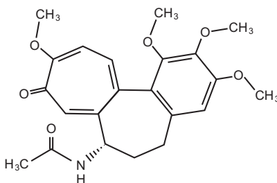
Colchicin
