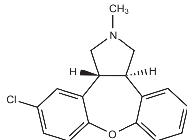
Asenapin
