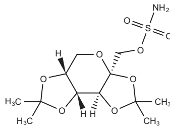
Topiramat
