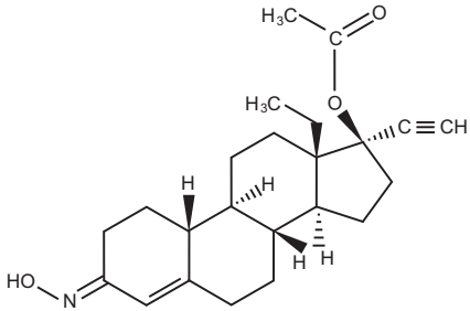
Norgestimat
