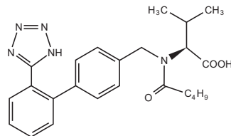
Valsartan
