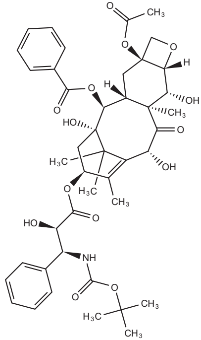
Docetaxel
