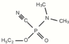
Tabun (Kampfstoff)
