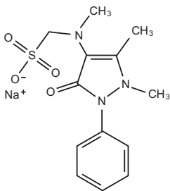
Metamizol
