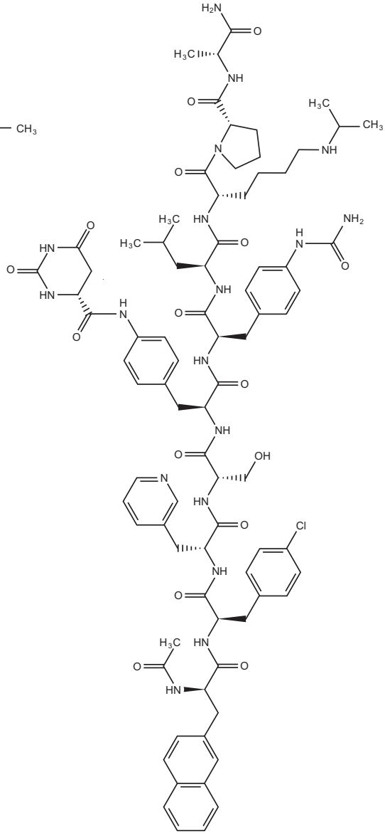
Degarelix
