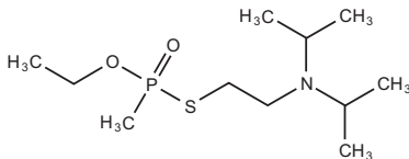
VX
