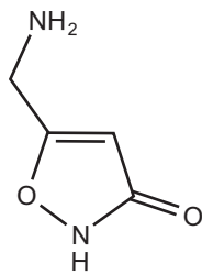
Muscimol
