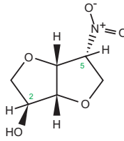
Isosorbidmononitrat
