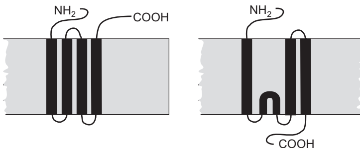
Abb. 9.11. Architektur des nACh-Kanals auf Muskelzellen (links) und auf Nervenzellen (rechts).
