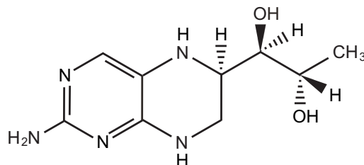
Sapropterin
