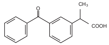
Ketoprofen
