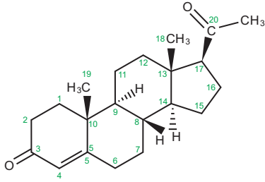
Progesteron
