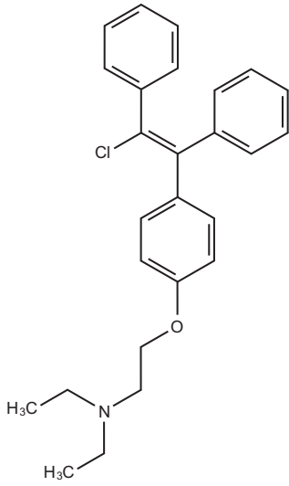
Clomifen
