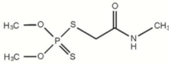
Dimethoat (Pestizid)
