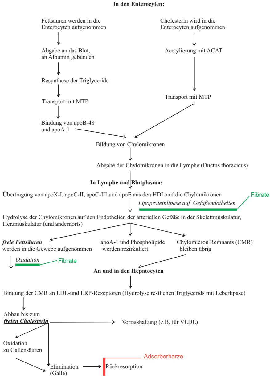
Abb. 32.2: Entstehen und Vergehen der Chylomikronen. Abkürzungen: ACAT Acetyl-Coenzym A: Cholesterin-O-acetyltransferase; apo Apoprotein; CMR chylomicron remnants; HDL high density lipoprotein; LDL low density lipoprotein; MTP microsomal triglycerid transport protein; NPC1L1 Niemann-Pick-like 1 protein; VLDL very low density lipoprotein. – Fibrate beschleunigen die Bildung freier Fettsäuren durch Vermehrung der Lipase und beschleunigen die Oxidation der in die Zellen aufgenommenen Fettsäuren. Adsorberharze hemmen die Rückresorption von Cholesterin und Gallensäuren.
