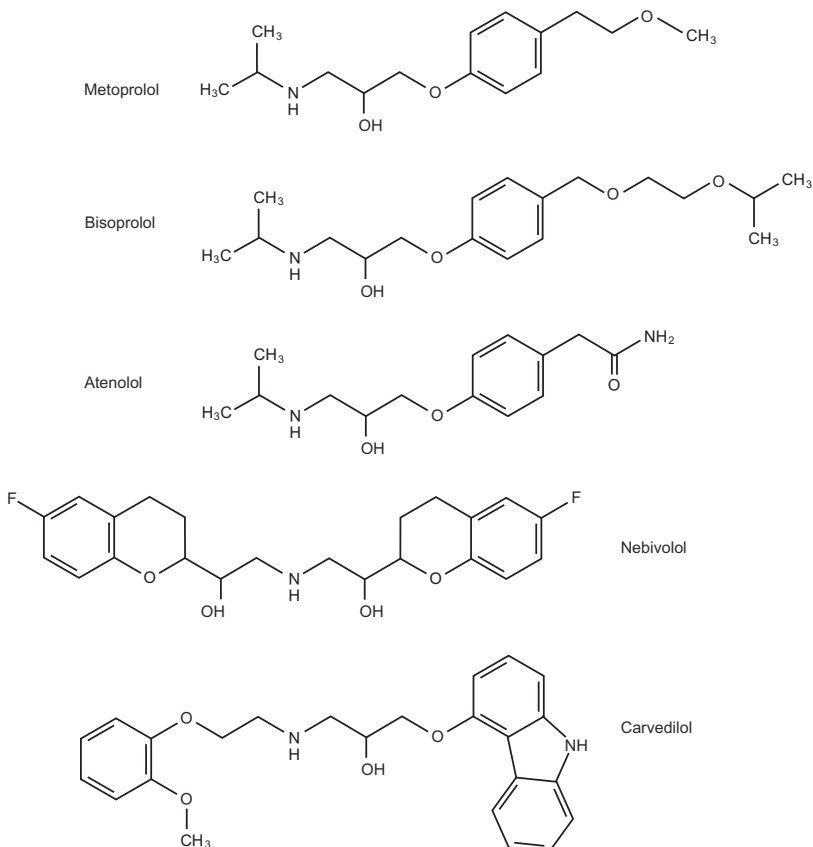
\beta_1 - Rezeptorantagonisten (Auswahl)
