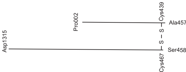
Abb. 64.3. Kettenstruktur von Botulinumtoxin A
