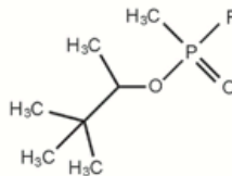
Soman (Kampfstoff)
