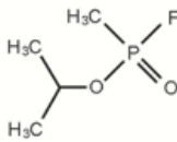
Sarin (Kampfstoff)
