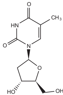
Telbivudin
