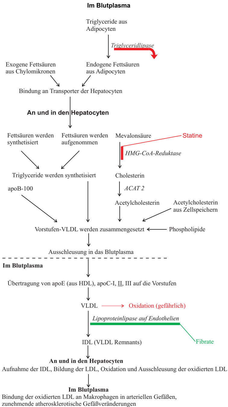
Abb. 32.3: Entstehen und Vergehen der VLDL. Abkürzungen: ACAT Acetyl-Coenzym A: Cholesterin-O-actyltransferase; apo Apoprotein; IDL intermediate density vesicles = VLDL remnants; LDL low density lipoprotein; MTP microsomal triglyce-
