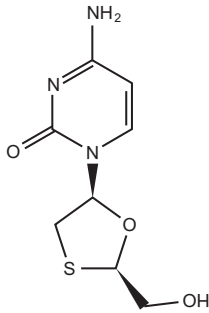
Lamivudin
