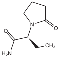
Levetiracetam
