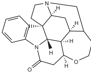
Strychnin
