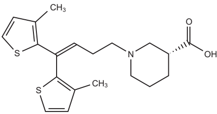
Tiagabin
