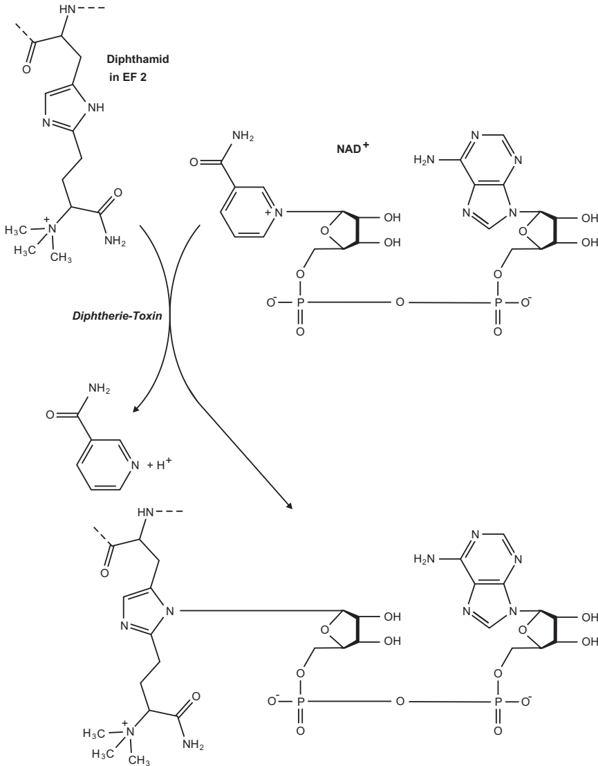
Abb. 111.2. Diphtherietoxin katalysiert die ADP-Ribosylierung der Aminosäure Diphthamid im Elongationsfaktor 2 (EF2).
