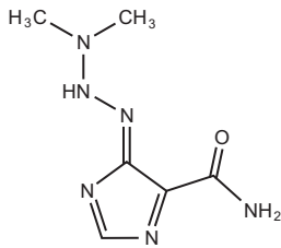
Dacarbazin
