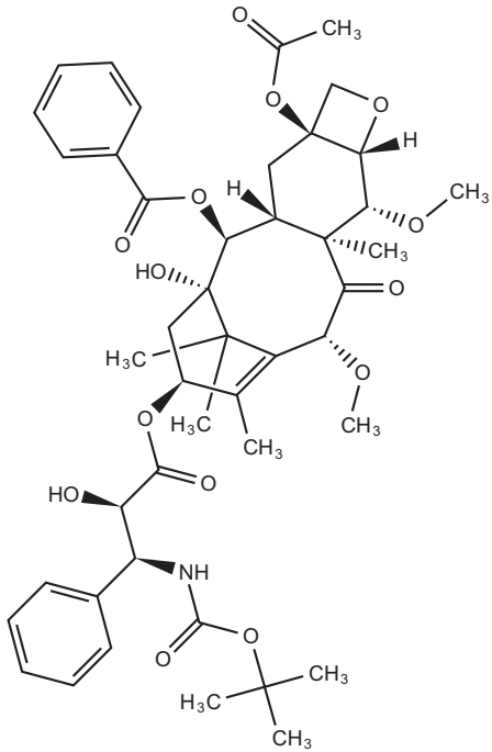
Cabazitaxel
