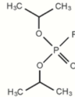
DFP (Reagenz)
