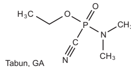
Tabun, GA
