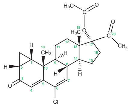
Cyproteronazetat
