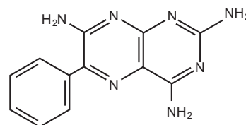
Triamteren
